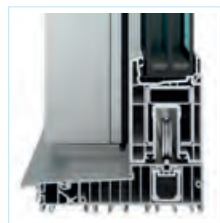
Práh s pojezdovým křídlem
