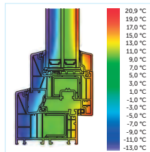
Průběh izoterm
