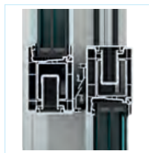
Průřez křídly
