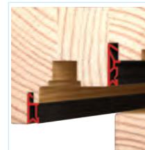
Systém těsnění
